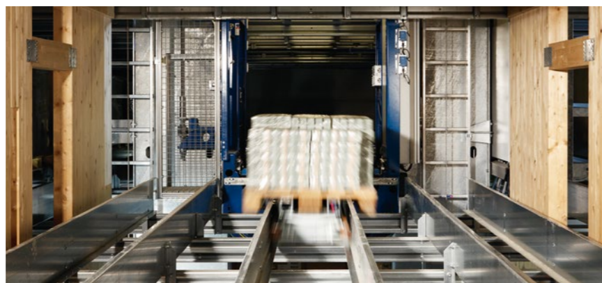
Einlagerung einer Palette mittels Längsshuttle in ein Fach des Holzregals. Für die innovative Konstruktion des Regals zeichnet der Holzbaupionier Kaufmann Bausysteme aus dem benachbarten Bregenzerwald verantwortlich – bewährter LTW-Partner bereits beim ersten Hochregallager aus Holz für die Salinen Austria.
